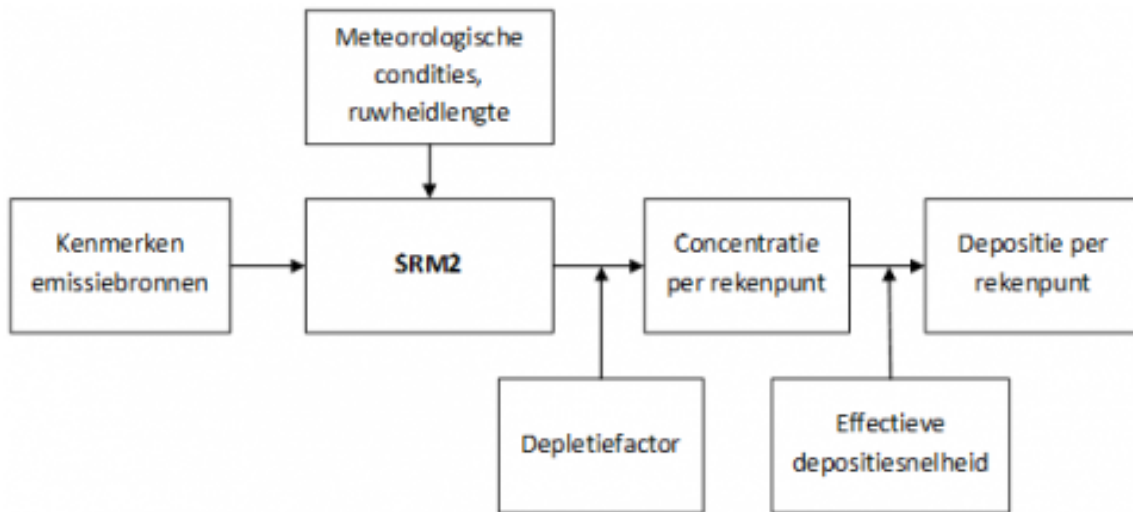
Figuur 23: Schematisch overzicht van de in- en uitvoer bij berekeningen met SRM-2
