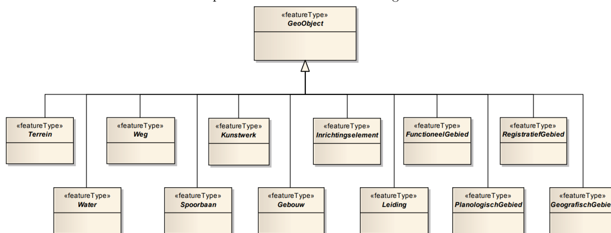
Figuur 70: UML Klassediagrammen
