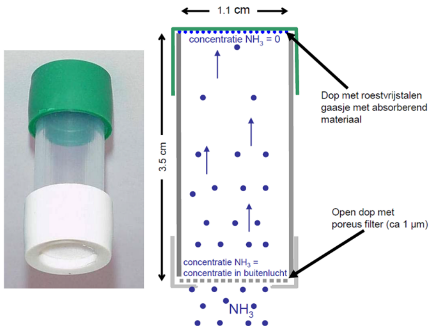
Figuur 5: Een Gradko-meetbuisje
